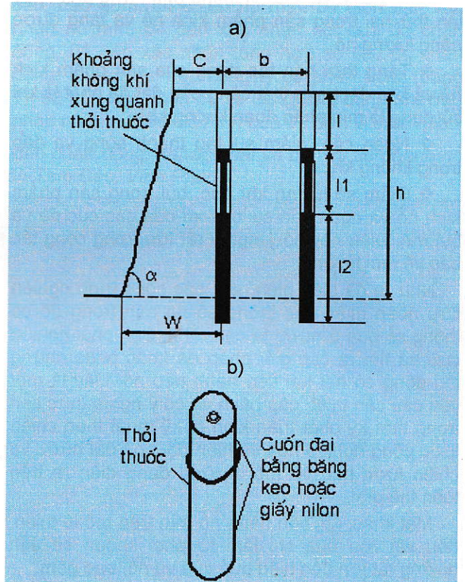
H.1. Sơ đồ cấu trúc lượng thuốc có đường kính khác nhau trong lỗ khoan: a - Cấu trúc lượng thuốc trong lỗ khoan; b - Cách tạo khoảng không khí xung quanh thối thuốc
