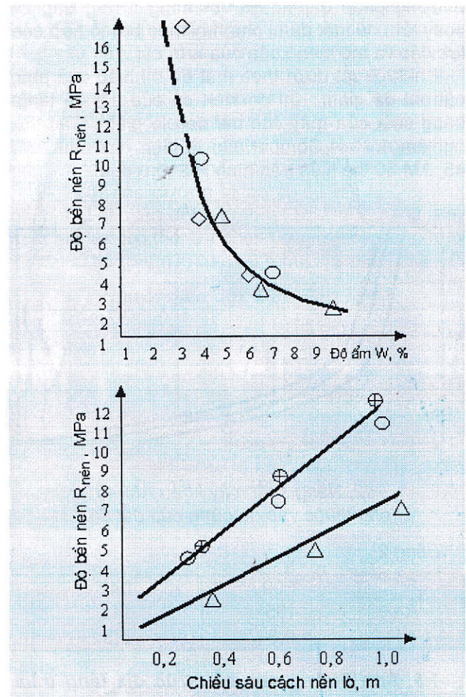
H.1. Ảnh hưởng của độ ẩm và chiều sâu nguyên khối đến độ bền của đá
