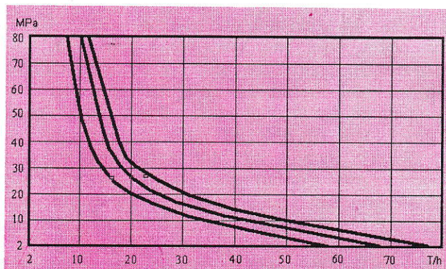
H.2. Năng suất máy khâu AM-45 phụ thuộc vào độ cứng của đất đá
