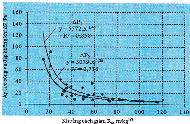
H.3. Sự phụ thuộc của áp lực sóng và đập không khí với khoảng cách giảm ( R_g ) khi tiến hành nổ mìn trong các mùa thu-đông ( \Delta P_1 ) và xuân-hạ ( \Delta P_2 )
