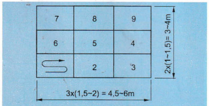
H.1. Trình tự và chia vùng phun trong thi công bê tông phun [1]: a - Phần nóc đường hầm; b - Phần tường đường hầm
