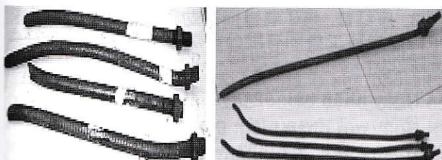
H.11. Vị trí đứt thân cốt neo tại phần giao giữa chất dính kết và đoạn tự do
