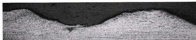
H.8. Nứt và bị han rỉ đáy chân ren
