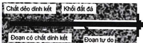
H.12. Cấu trúc trong lỗ khoan thân cốt neo thép đặc có chất dẻo dính kết
