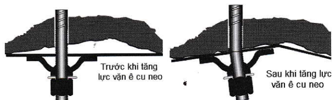
H.9. Hiện tượng thanh neo bị gãy gập khi tăng lực vận đai ốc neo
