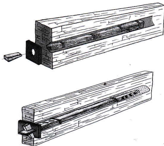
H.1. Thân cốt neo bằng tre và gỗ
