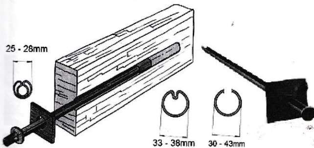
H.3. Thân cốt neo bằng thép ống
