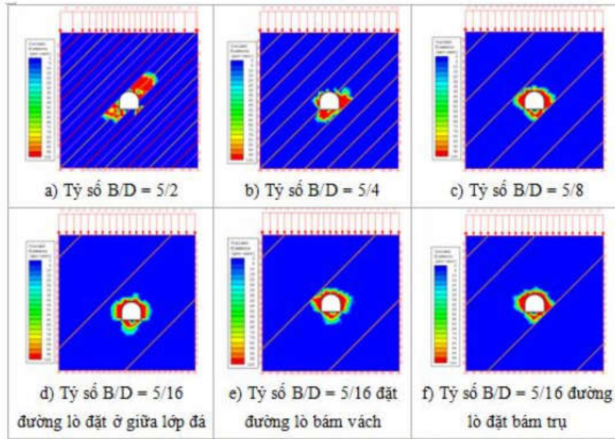
H.4. Mô phỏng sự xuất hiện vùng phá hủy xung quang đường lò nằm trong các lớp đất đá dốc (Thành tựu bước đầu thiết kế giếng đứng của các nhà khoa học Việt Nam,...)
