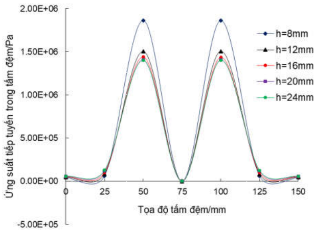
H.5. Đường cong phân bố ứng suất tiếp tuyến ứng với các chiều dày tấm đệm
