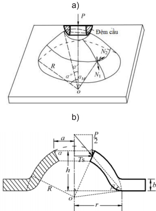
Hình 2. Mô hình tính toán chịu lực của tấm đệm cầu a) Mô hình chịu lực của tấm đệm cầu, b) mặt cắt hình học tấm đệm cầu
