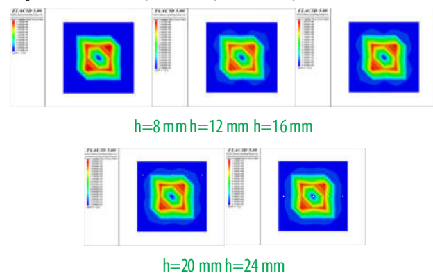
H.4. Phân bố ứng suất tiếp tuyến trên tấm đệm ứng với các chiều dày
