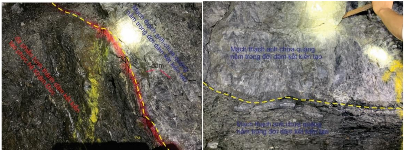
Hình 2. Mạch thạch anh xuyên cắt đới dăm kết kiến tạo trong đá phiến phức hệ Khâm Đức (a), quặng nằm chính hợp trong cấu tạo phiến trong lò khai thác quặng khu vực Bãi Giỏ (b) thuộc mỏ Phước Sơn
