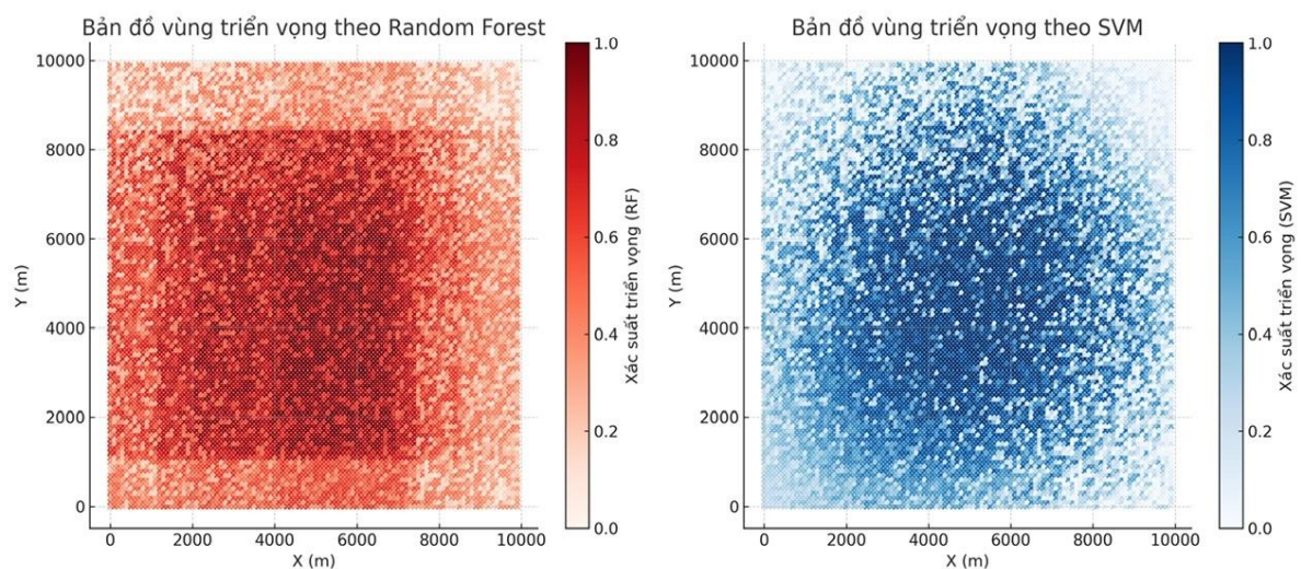
Hình 2. Minh họa cho phần Mô hình Machine Learning (RF & SVM)
